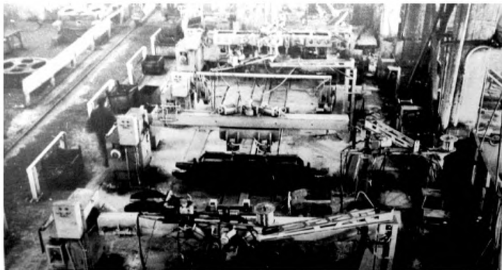
Конвейерная линия сборки гусениц экскаватора
