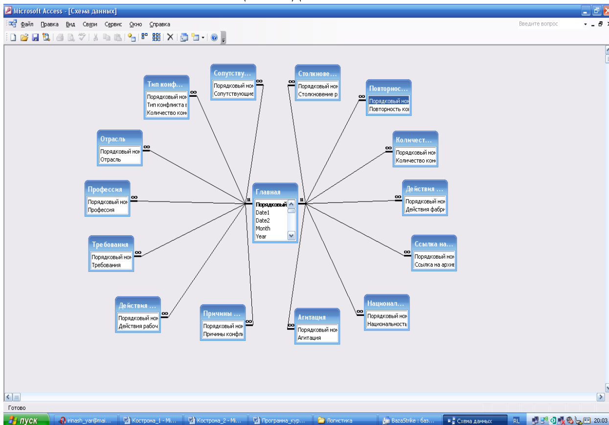
Рис.1. Схема связи таблиц базы данных
