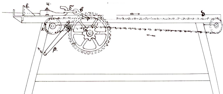
Рис. 2. Схема волочильной доски из металла
