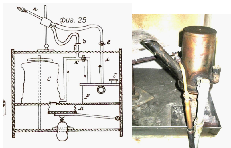
Рис. 3. Паяльные устройства
